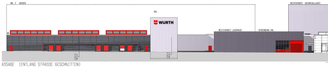
2D-Ansicht des Erweiterungsbaus (rechts bestehendes Lagergebäude)
